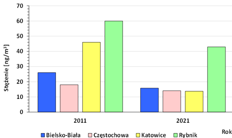
Rycina 31. Zmiany stężenia benzo( \alpha )pirenu ( B\alpha P ) w pyłach frakcji PM_{10} w powietrzu (w ng/m^3 ) odnotowane w głównych miastach subregionów w roku 2011 i 2021 – stężenie średnioroczne (A) i stężenie maksymalne (B) odnotowane w roku 2011 i 2021. Na podstawie: GIOŚ (2022).
