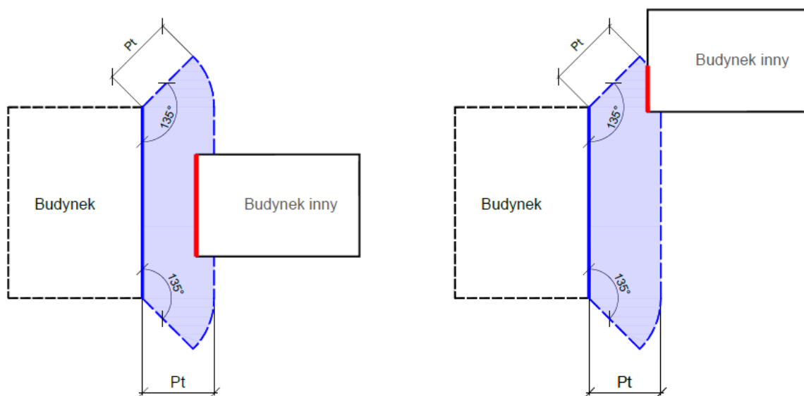
Rys. 1. Wyznaczanie pasa terenu wokół ściany zewnętrznej budynku – § 283 ust. 11.
