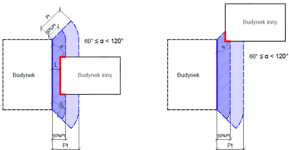
Rys. 2 Wyznaczanie pasa terenu wokół ściany zewnętrznej budynku dla ścian pod kątem innego budynku – § 283 ust. 11 i 12.
