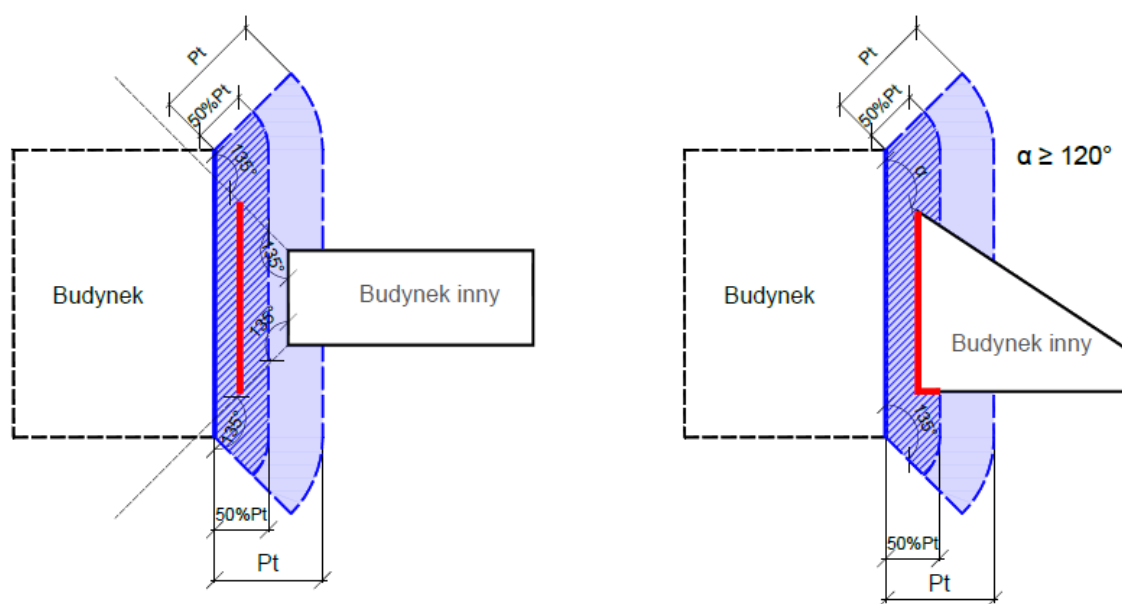
Rys. 3. Wyznaczanie pasa terenu wokół ściany zewnętrznej budynku przy zastosowaniu ściany oddzielenia przeciwpożarowego oraz dla ściany pod kątem – § 283 ust. 11–13.
