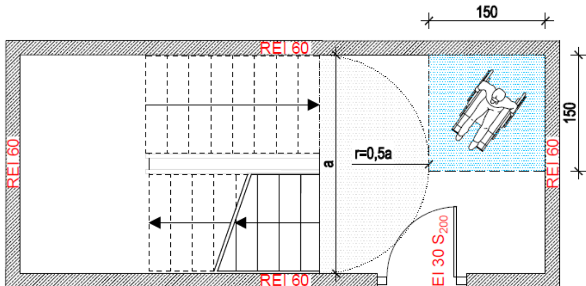
Rys. 1. Miejsce oczekiwania na ewakuację dla osób niepełnosprawnych, na spoczniku prostokątnym.
