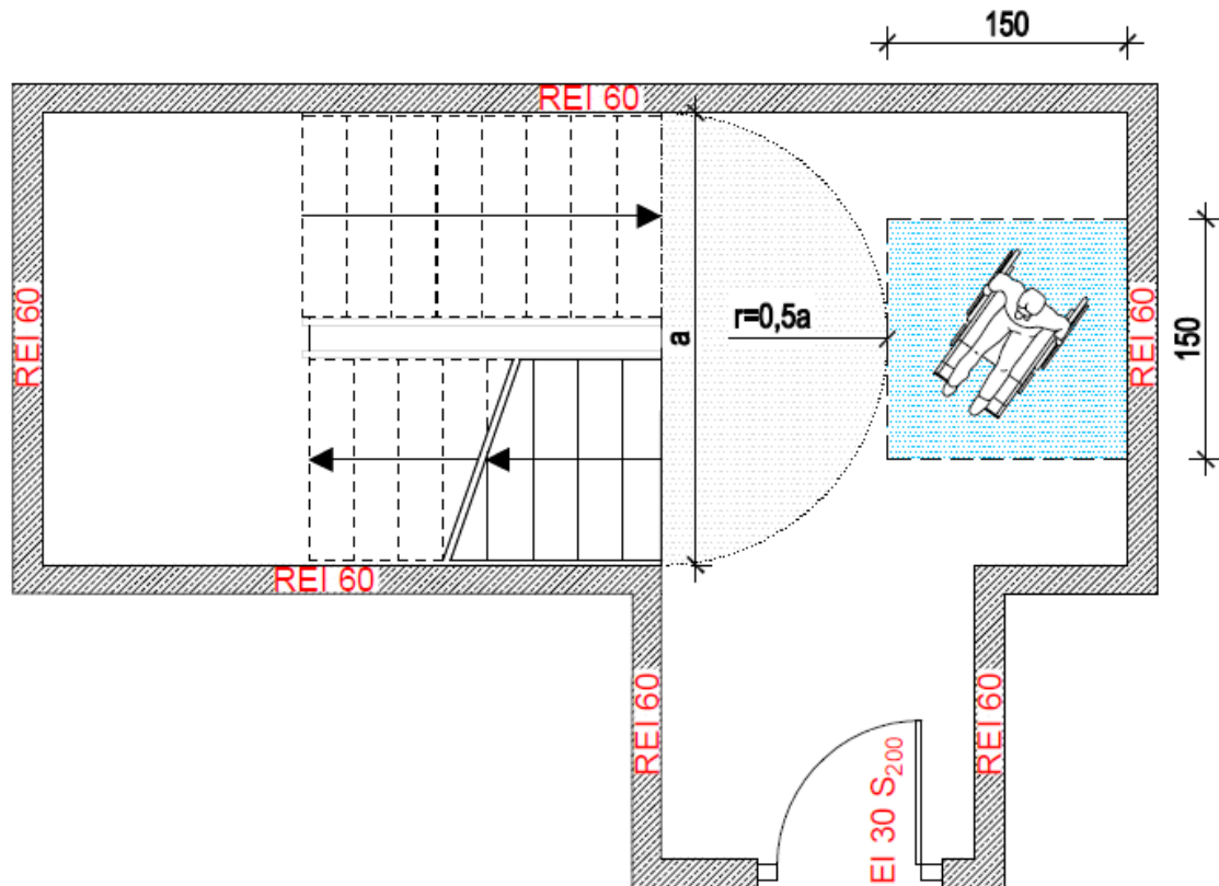
Rys. 3. Miejsca oczekiwania na ewakuację dla osób niepełnosprawnych, na spoczniku z wnękami.
