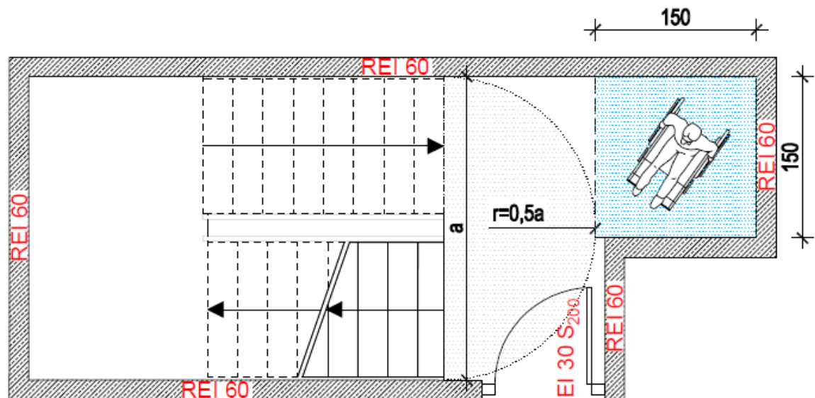
Rys. 2. Miejsce oczekiwania na ewakuację dla osób niepełnosprawnych, na spoczniku z wnęką.
