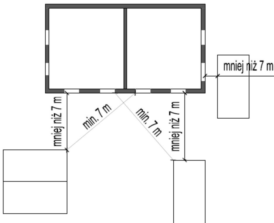
Rys. 4. Odległość od okna lub elementu doświetlającego pomieszczenia przeznaczonego na stały pobyt ludzi w budynku mieszkalnym jednorodzinnym w przypadku jednego albo dwóch stanowisk postojowych dla samochodów osobowych przypadających na jeden lokal mieszkalny w tym budynku – § 16 ust. 6.
