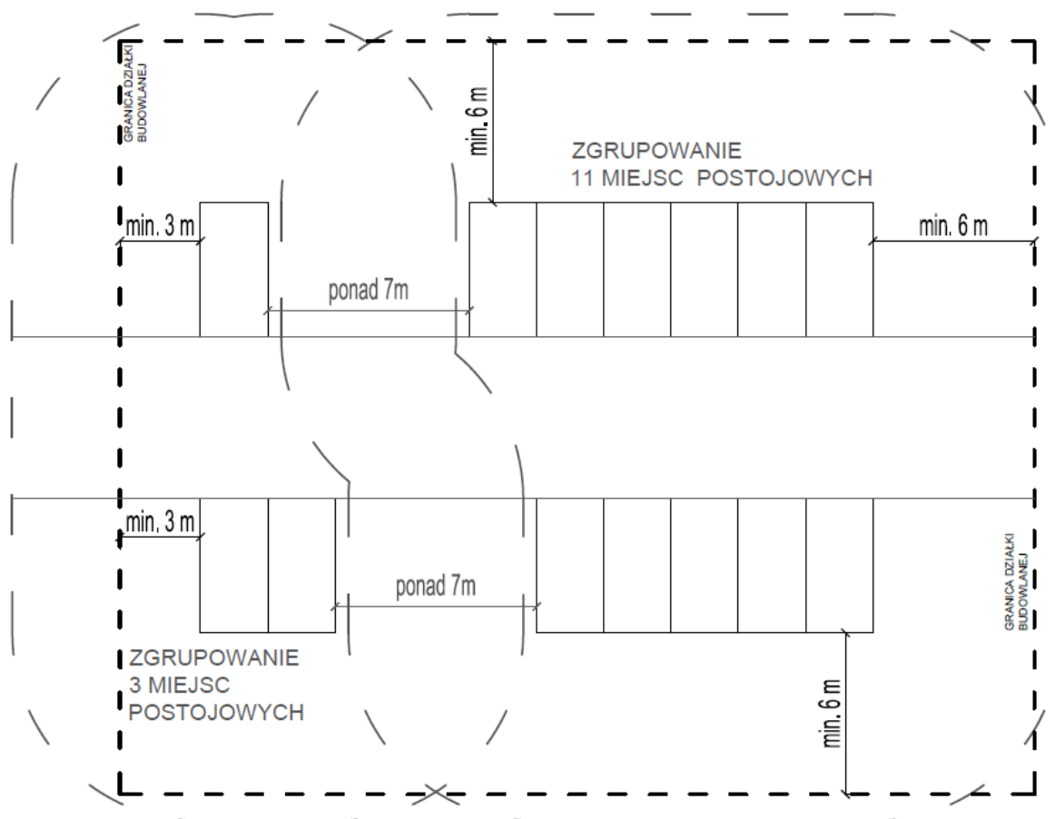
Rys. 2. Odległość od granicy tej działki budowlanej – § 16 ust. 2 pkt 1.
