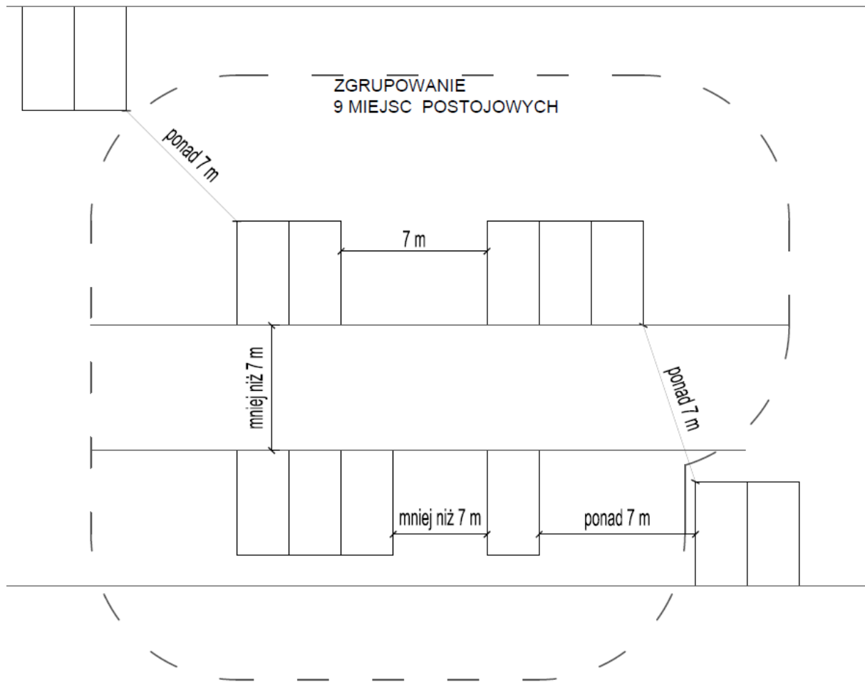
Rys. 3. Odległość pomiędzy poszczególnymi stanowiskami postojowymi tworzącymi zgrupowania w obrębie działki budowlanej – § 16 ust. 3.
