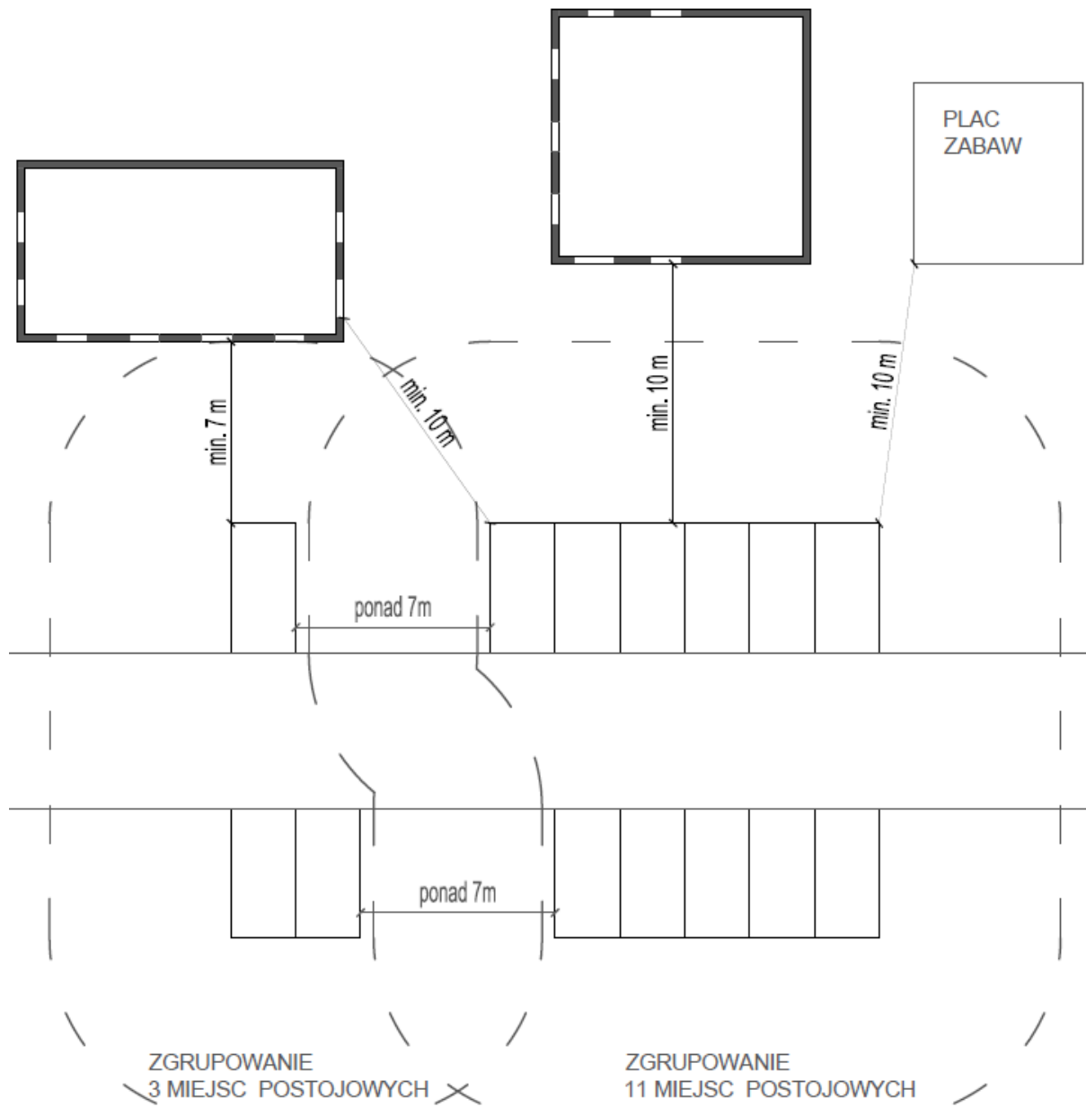
Rys. 1. Odległość od placu zabaw dla dzieci, okna lub elementu doświetlającego pomieszczenia przeznaczonego na stały pobyt ludzi – § 16 ust. 1 pkt 1.
