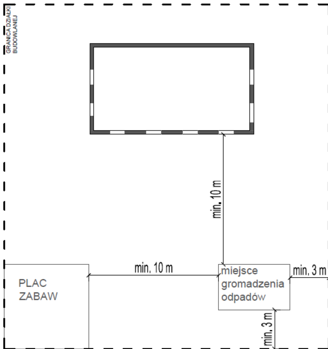
Rys. 1. Odległość od okna lub drzwi pomieszczenia przeznaczonego na pobyt ludzi; od granicy tej działki budowlanej; od placu zabaw dla dzieci – § 20 ust. 1.
