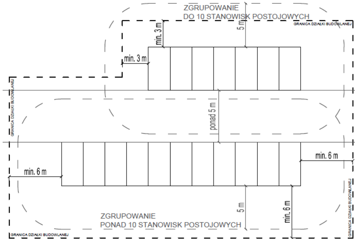
Rys. 2. Minimalna odległość stanowiska postojowego i zgrupowania stanowisk postojowych od granicy tej działki budowlanej – § 16 ust. 2 pkt 1 oraz § 16 ust. 3.
