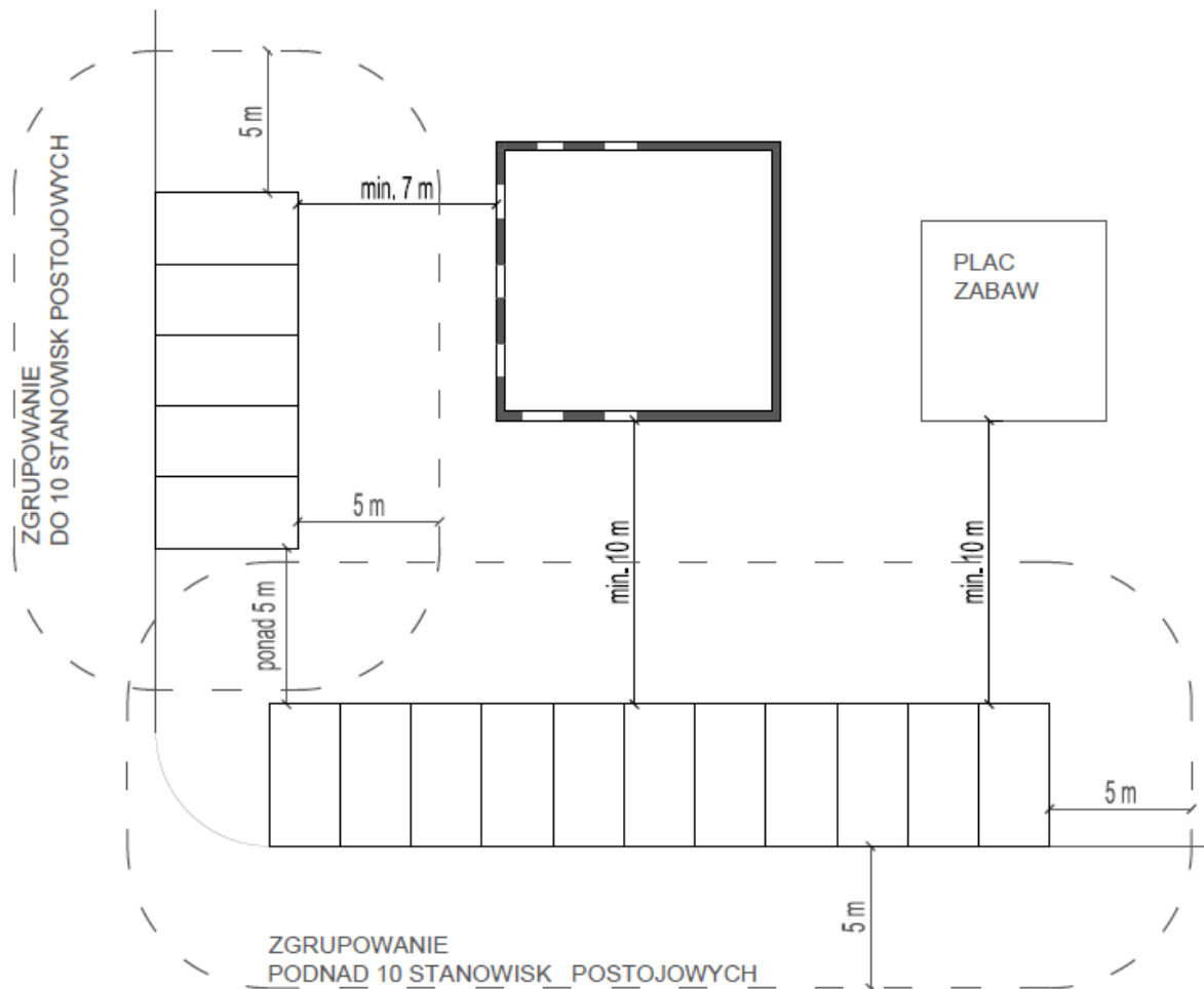
Rys. 1. Minimalna odległość stanowiska postojowego i zgrupowania stanowisk postojowych od placu zabaw dla dzieci, okna lub elementu doświetlającego pomieszczenia przeznaczonego na stały pobyt ludzi – § 16 ust. 1 pkt 1 oraz § 16 ust. 3.
