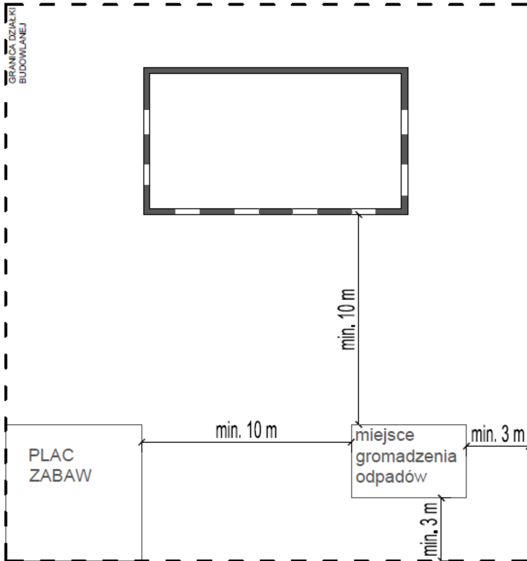
Rys. Minimalna odległość miejsca do gromadzenia odpadów stałych od: okna lub drzwi pomieszczenia przeznaczonego na pobyt ludzi, granicy tej działki budowlanej, placu zabaw dla dzieci – § 20 ust. 1.
